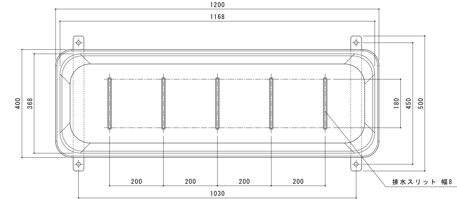
上面図
