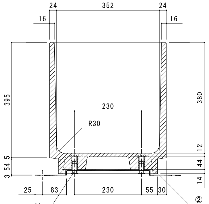
A-A' 断面図
