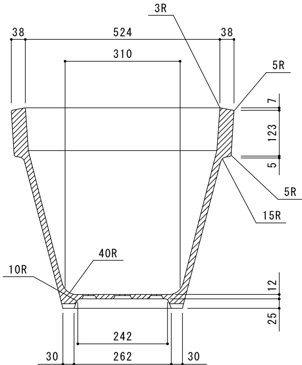
A-A' 断面図
