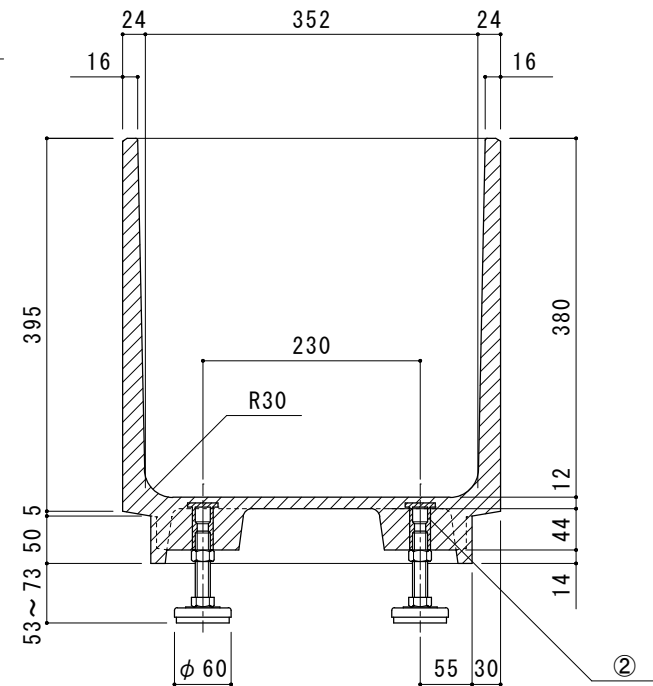
A-A'断面図
