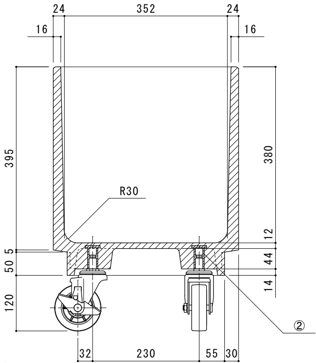
A-A'断面図
