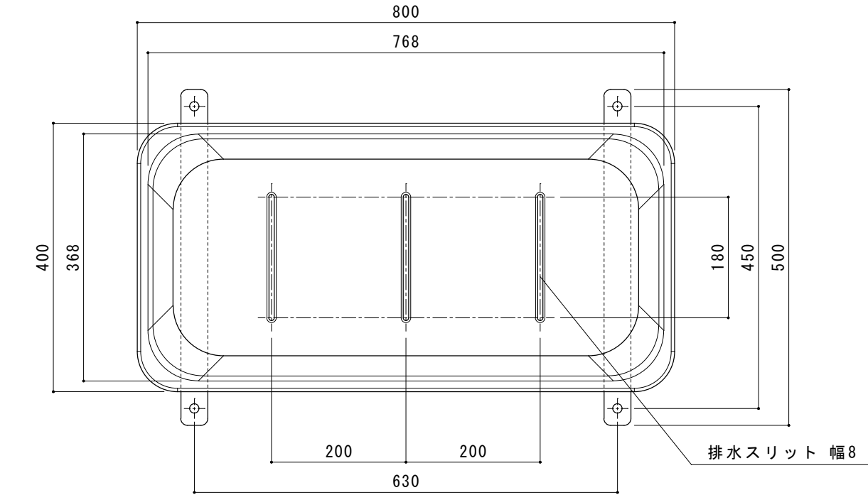
上面図
