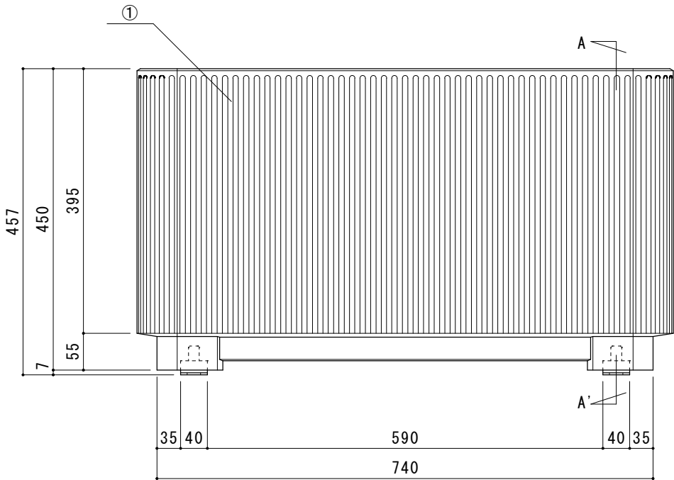
正面図
