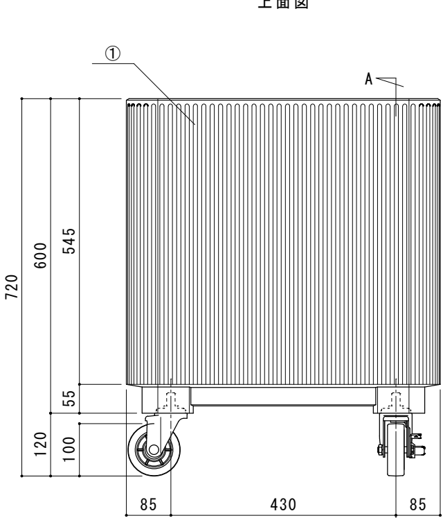
正面図
