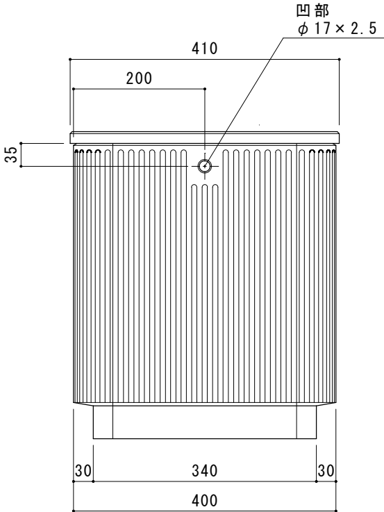
側面図
