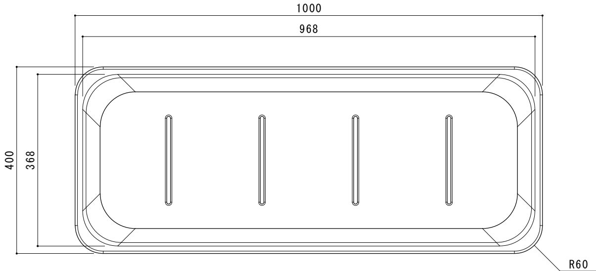
上面図
