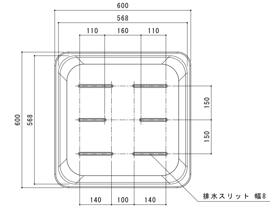
上面図
