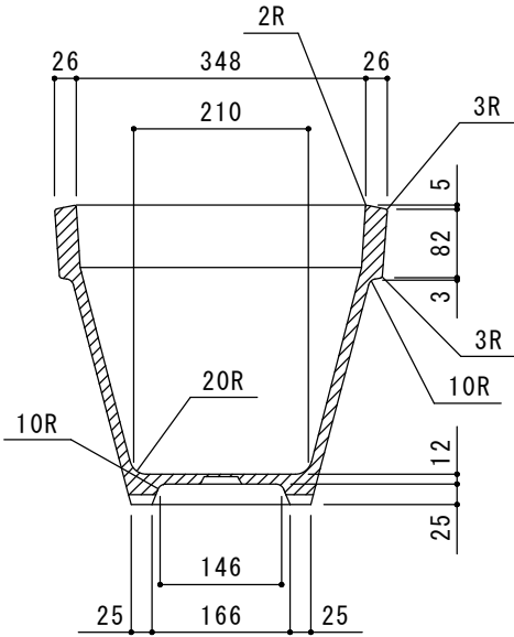
A-A' 断面図
