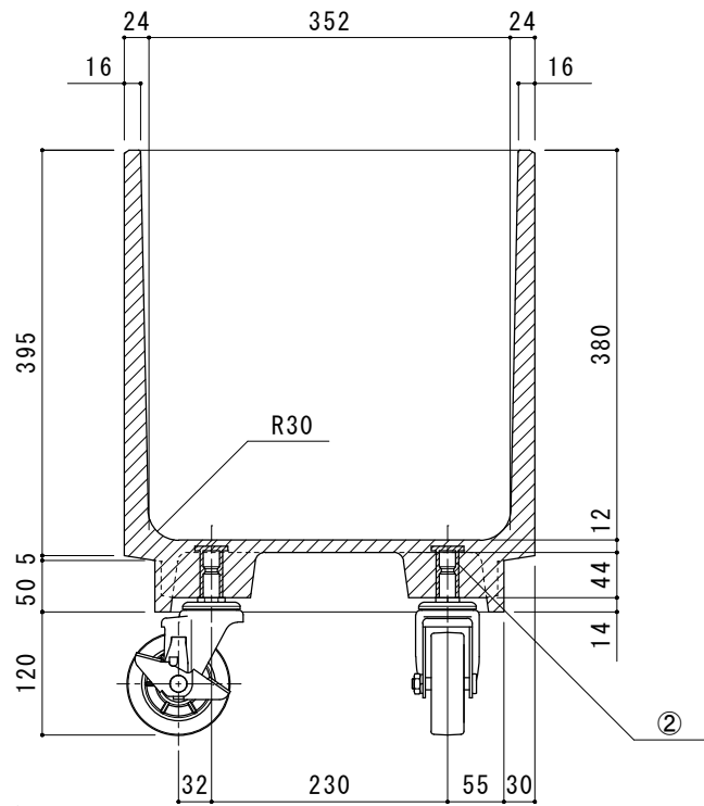
A-A'断面図
