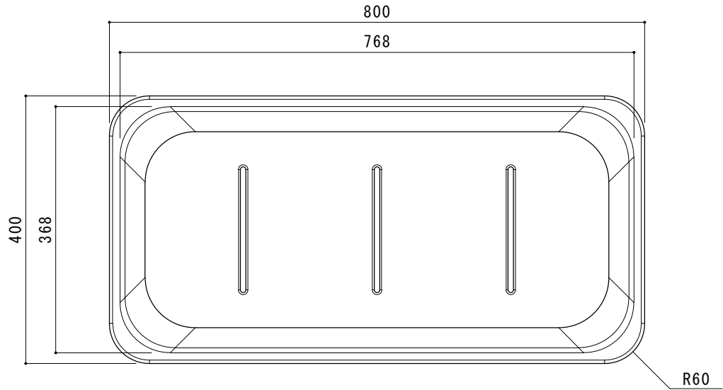
上面図
