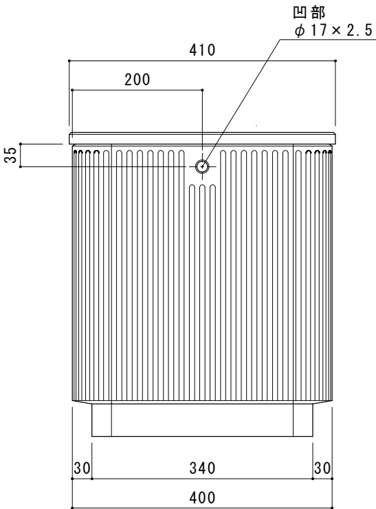
側面図
