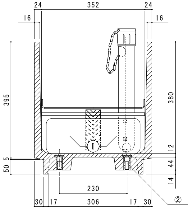
A-A' 断面図
