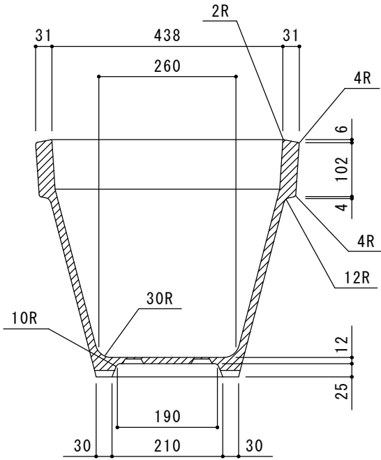
A-A' 断面図
