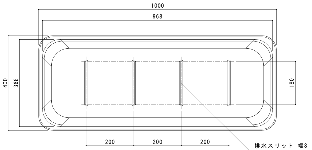
上面図
