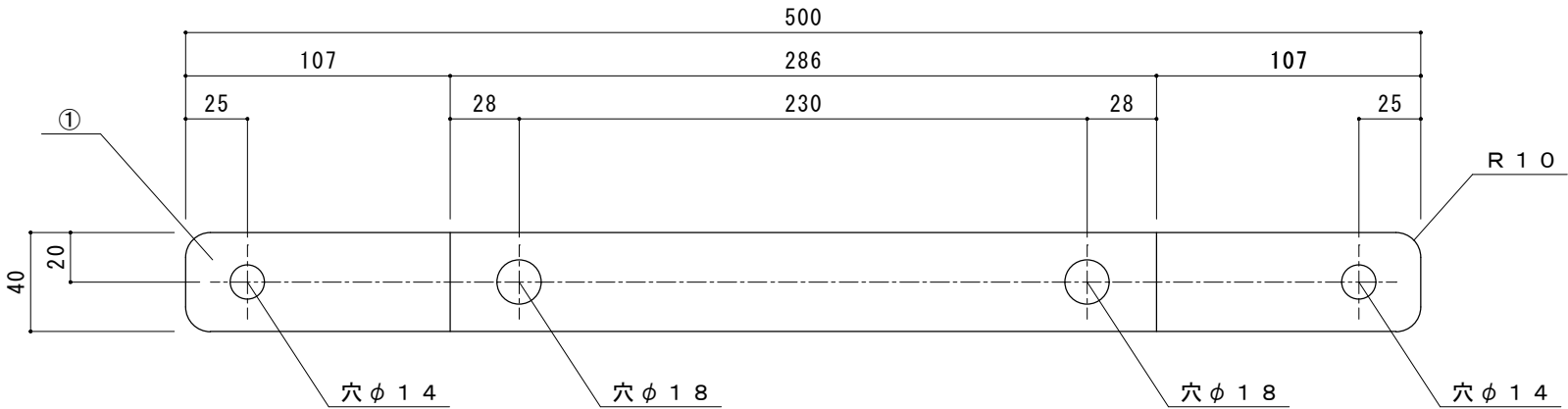
上面図
