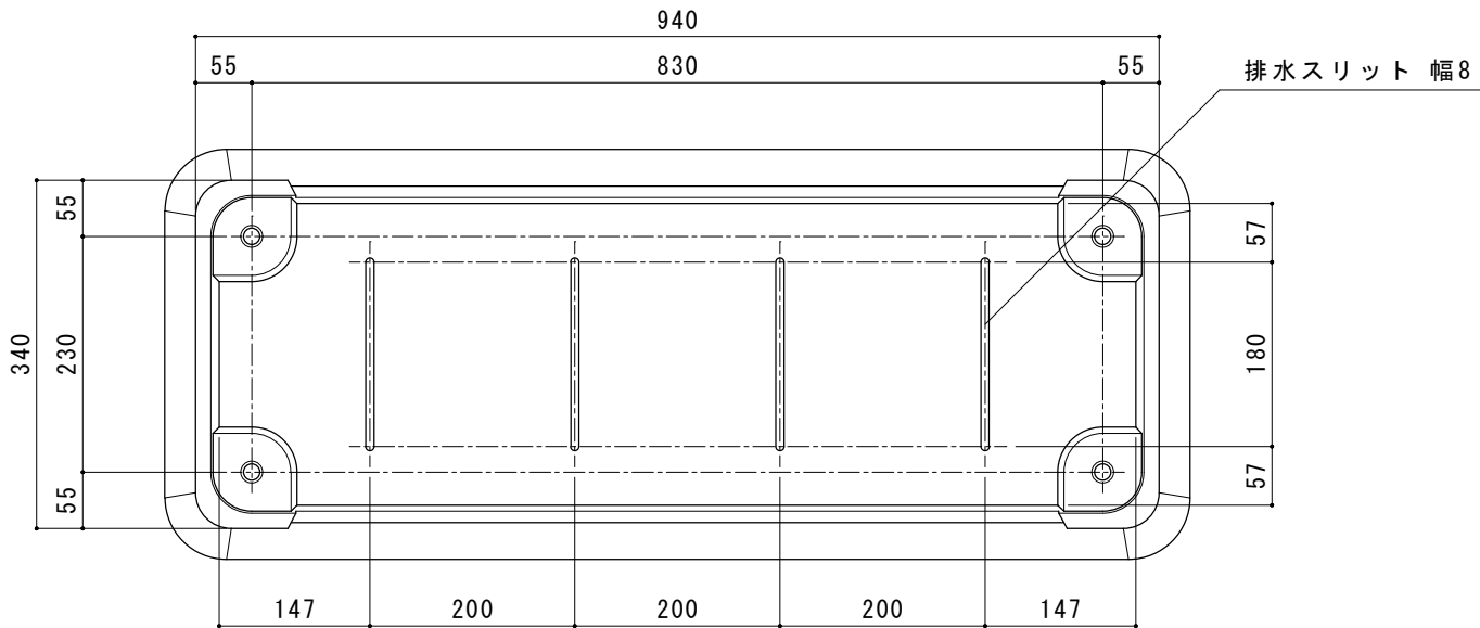
底面図
