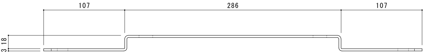
正面図
