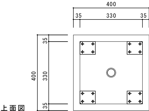
上面図
