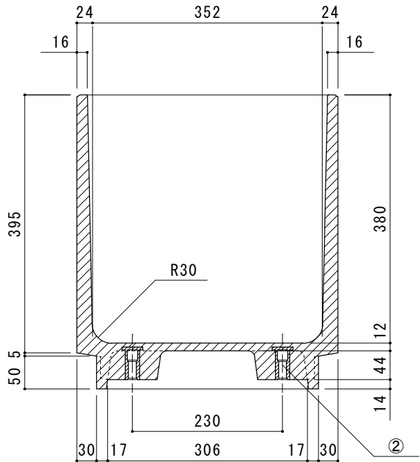
A-A' 断面図
