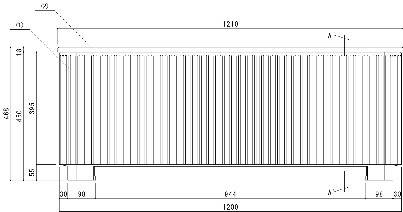
正面図
