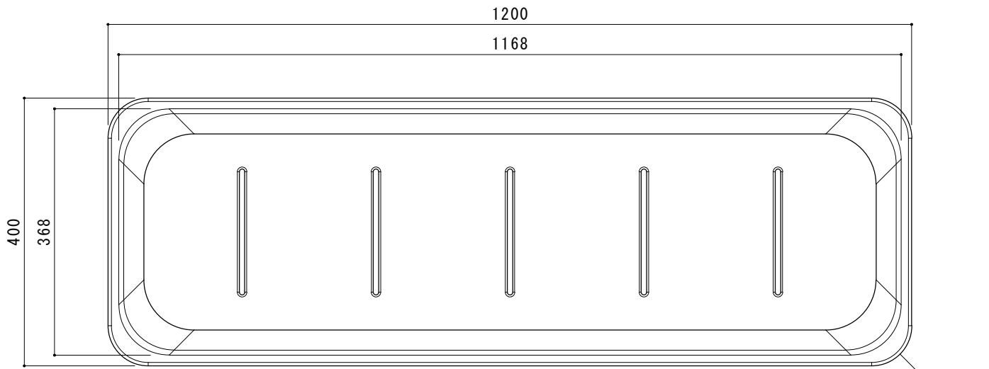
上面図
