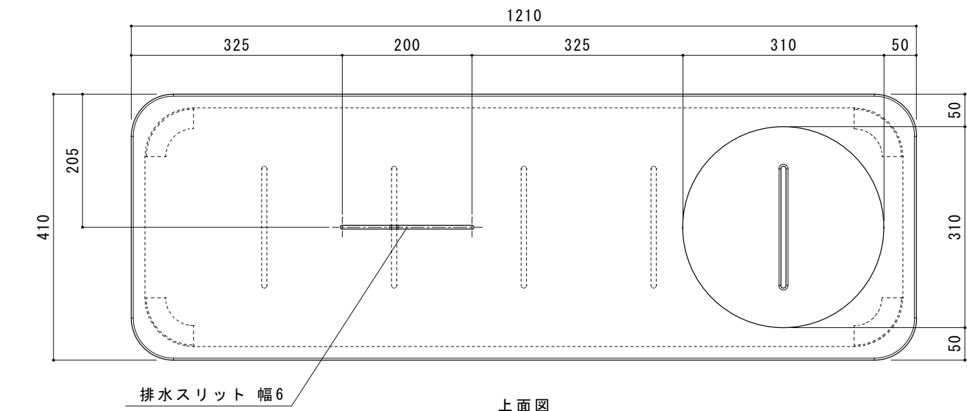
上面図
