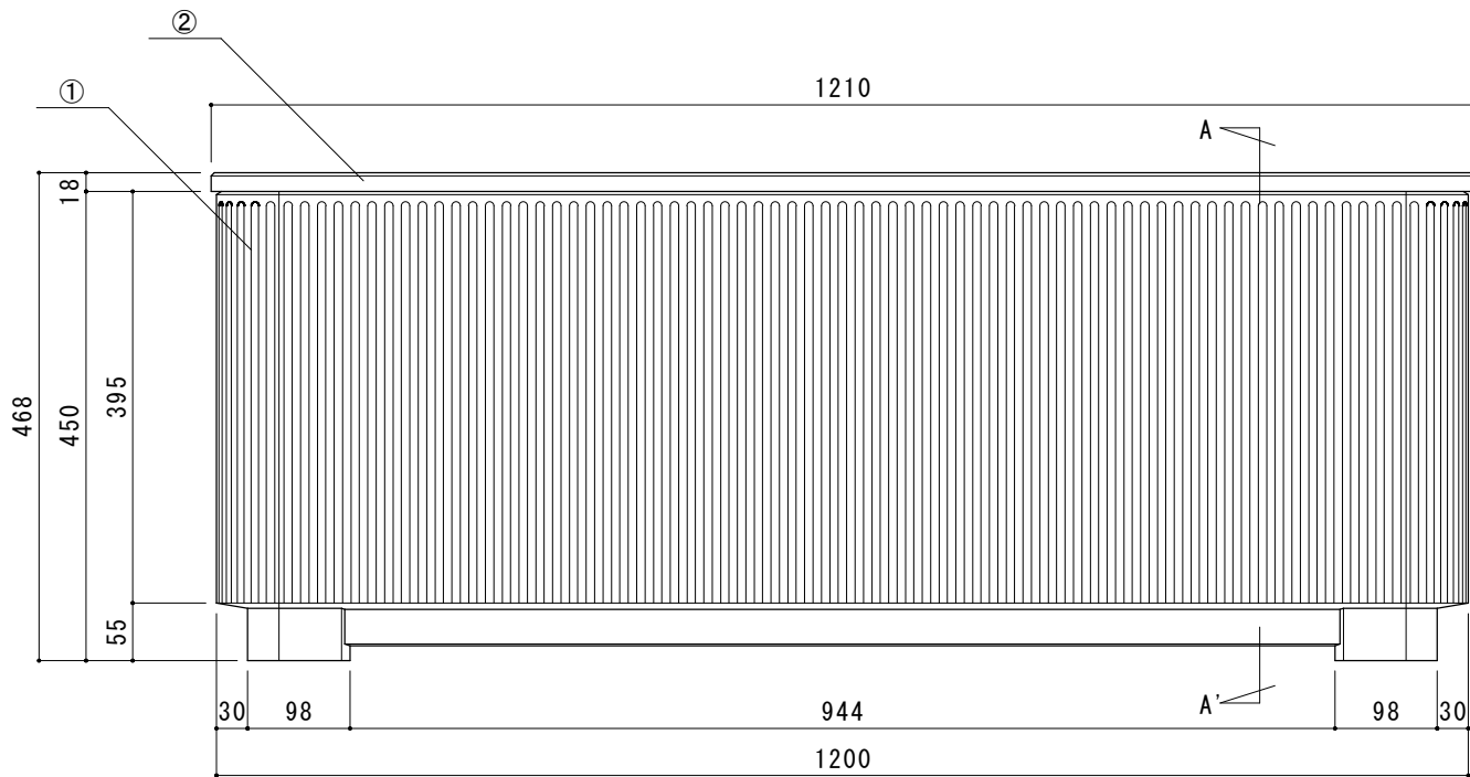
正面図
