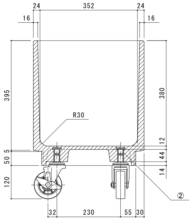
A-A'断面図
