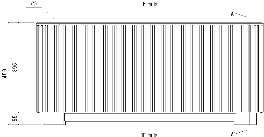
正面図
