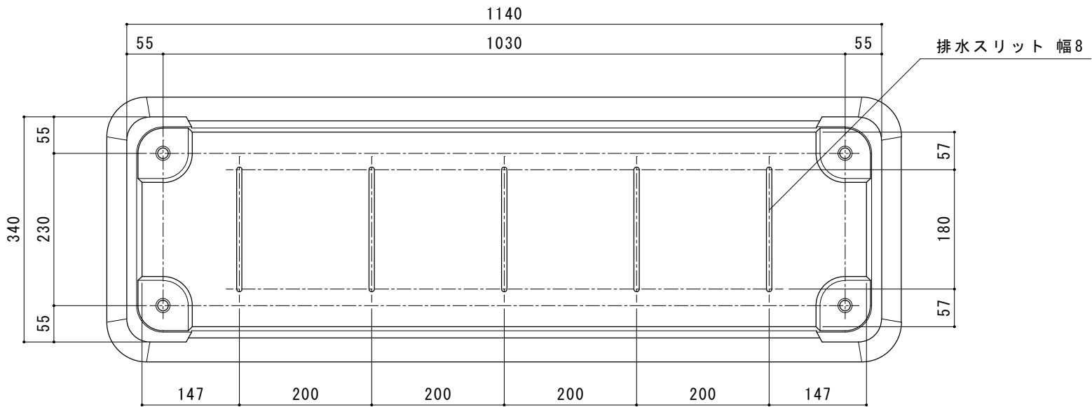
底面図
