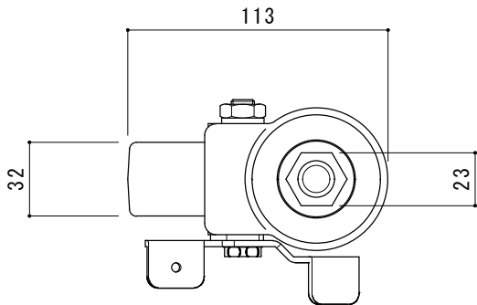
上面図
