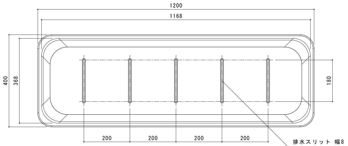
上面図
