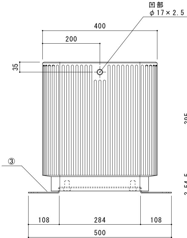
側面図
