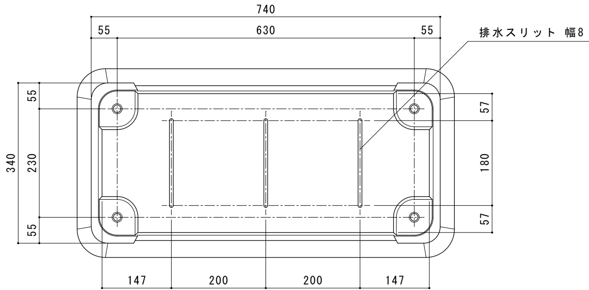
底面図
