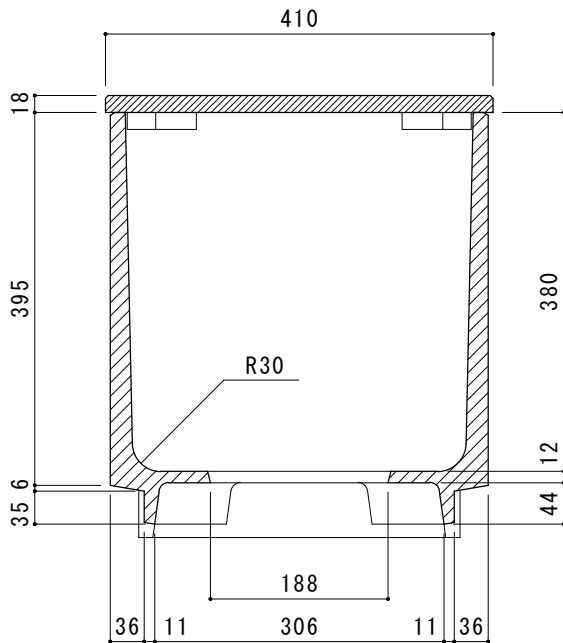
A-A' 断面図
