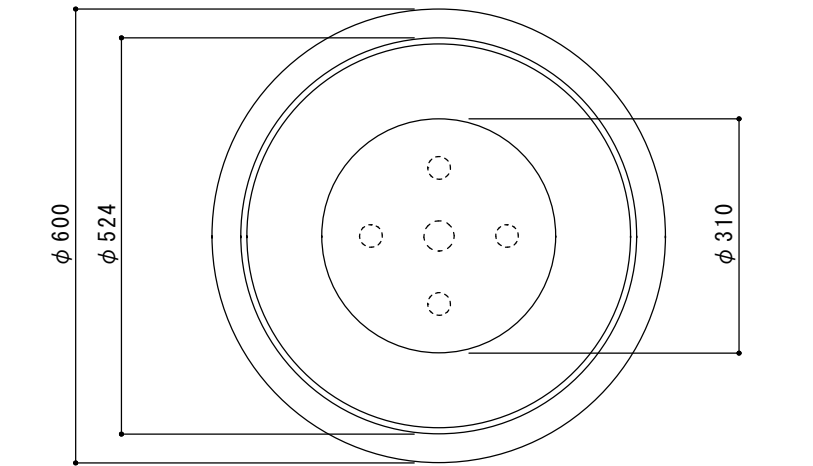
上面図
