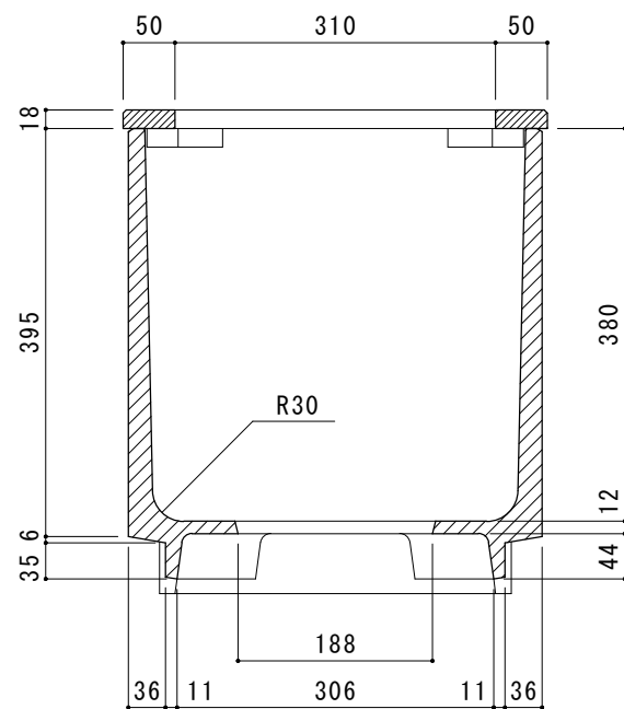
A-A' 断面図
