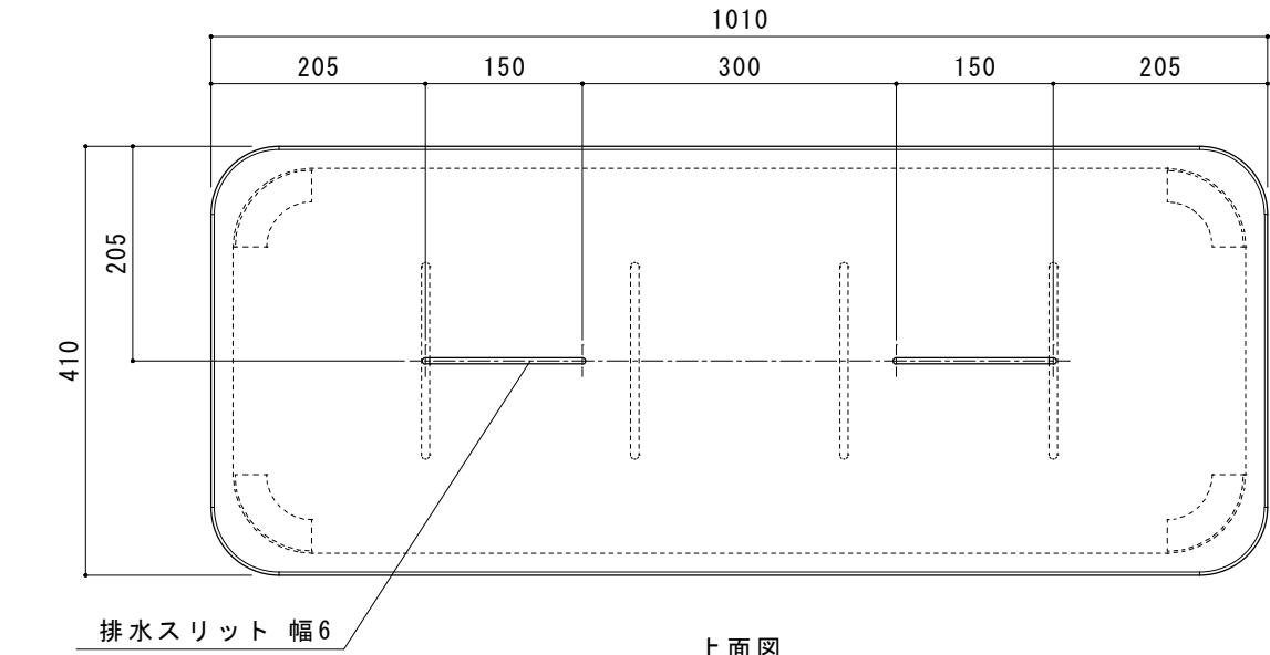
上面図
