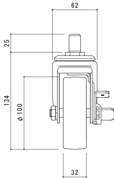
側面図
