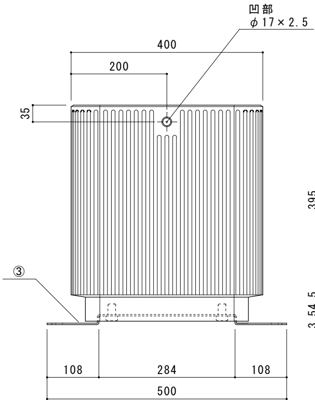
側面図
