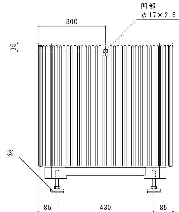
側面図
