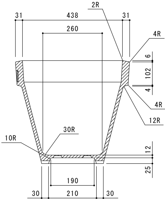
A-A' 断面図
