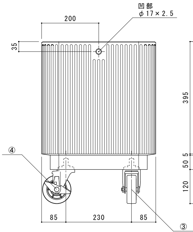
側面図
