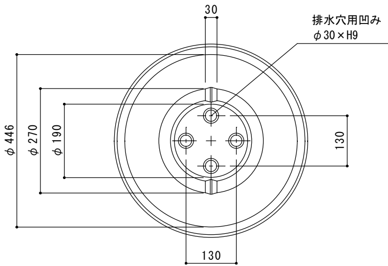
底面図
