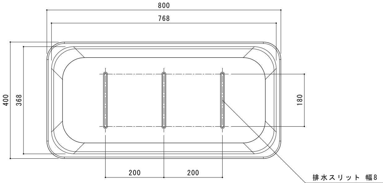
上面図
