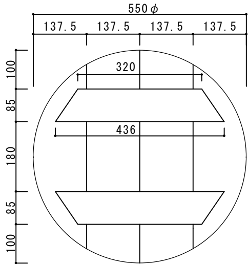
座部底面図
