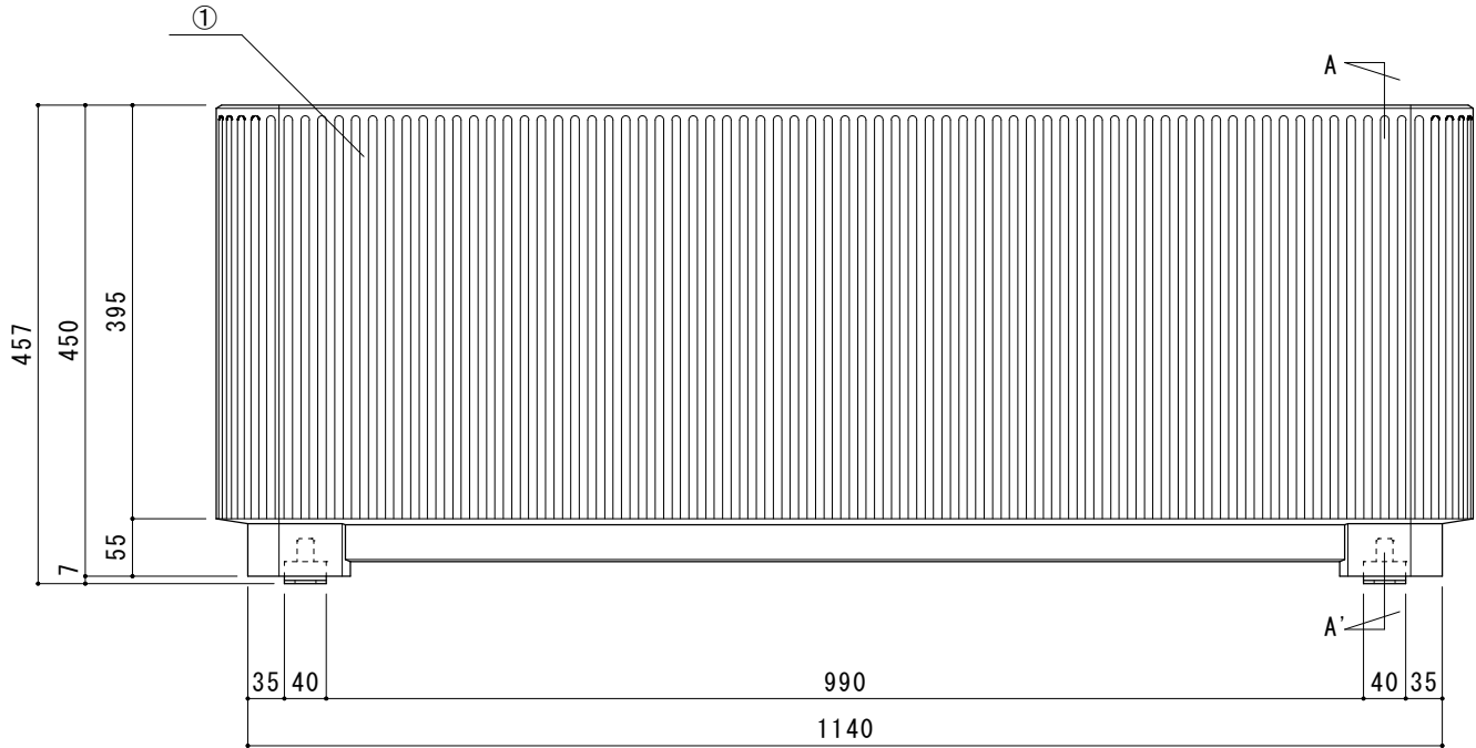
正面図
