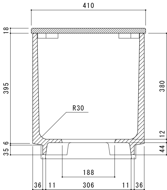
A-A'断面図
