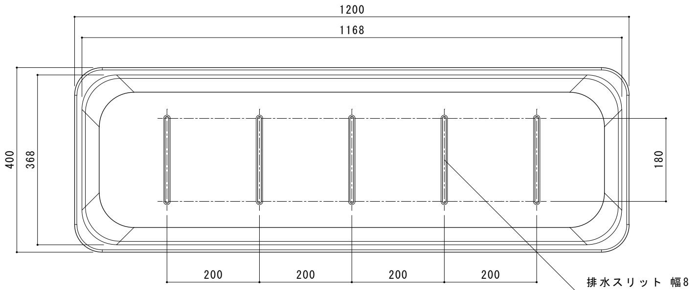
上面図
