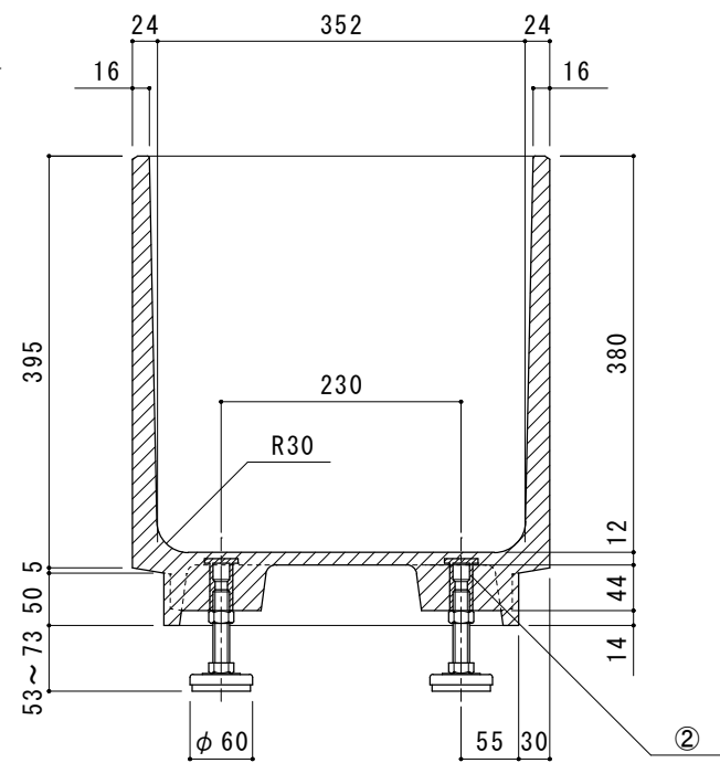
A-A'断面図
