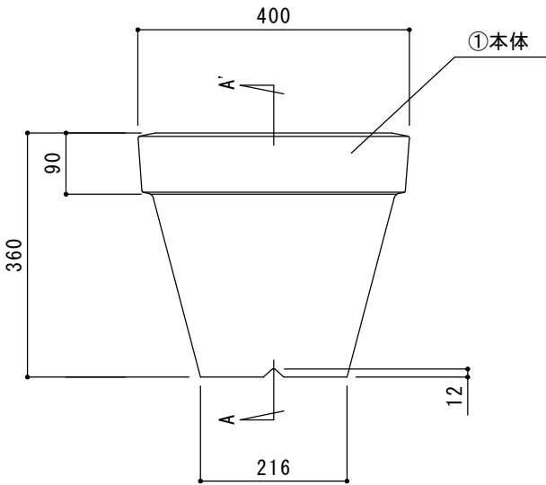
立面図
