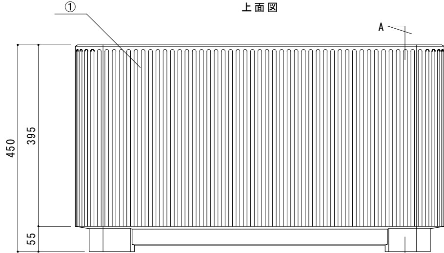
正面図
