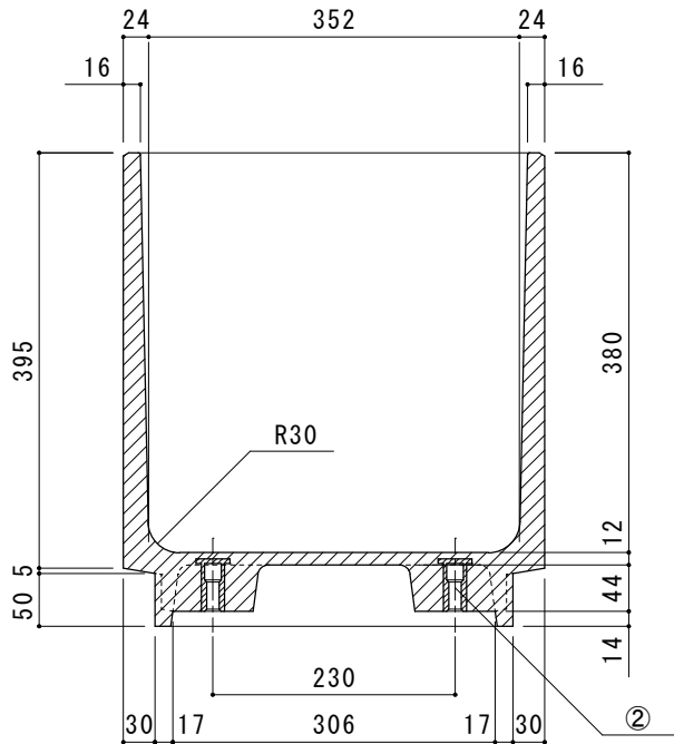
A-A' 断面図
