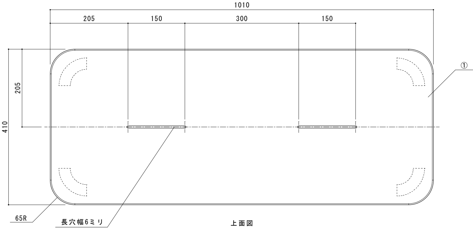
上面図
