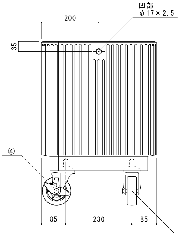
側面図
