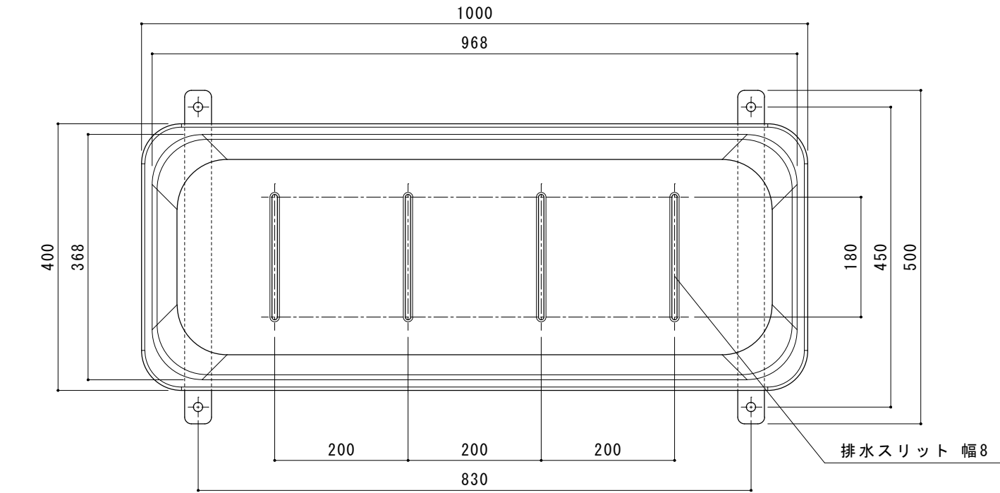
上面図
