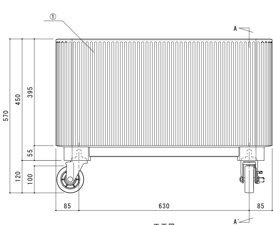
正面図
