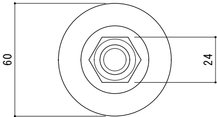
上面図
