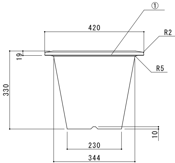
立面図
