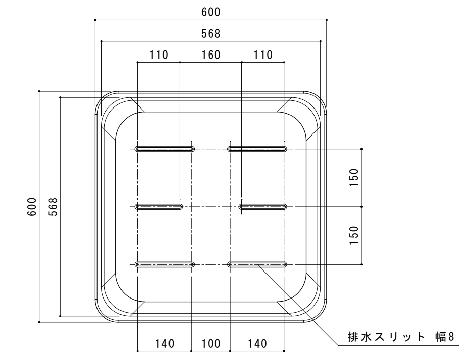
上面図
