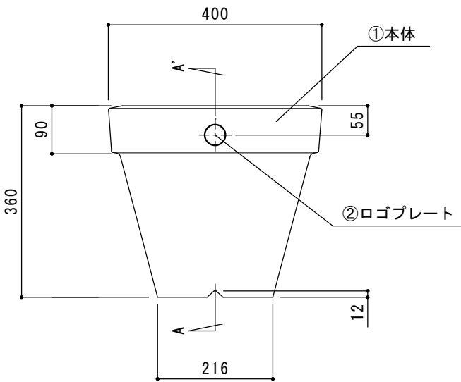
立面図
