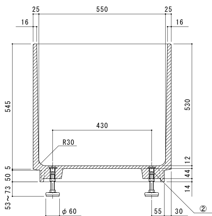
A-A'断面図
