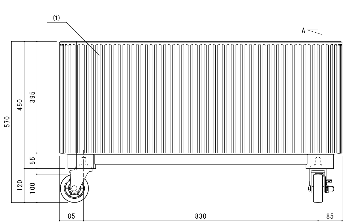
正面図
