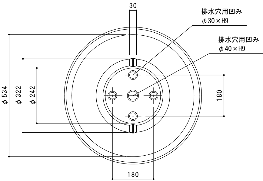
底面図
