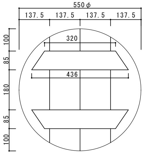
座部底面図
