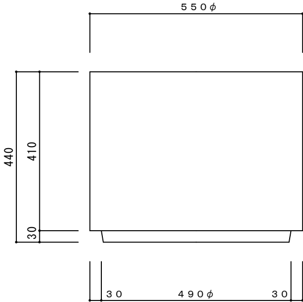
正面図
