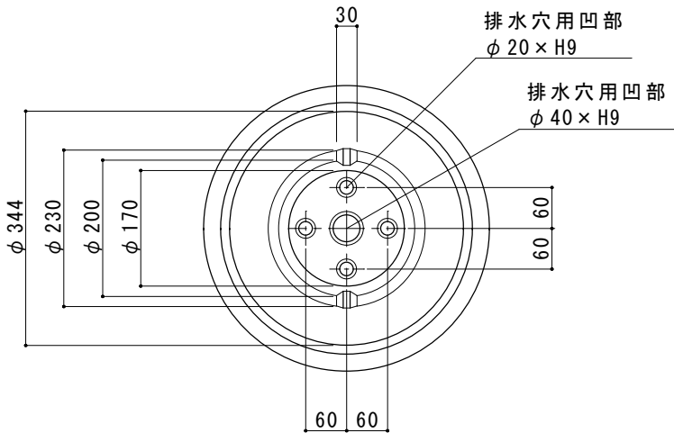
底面図
